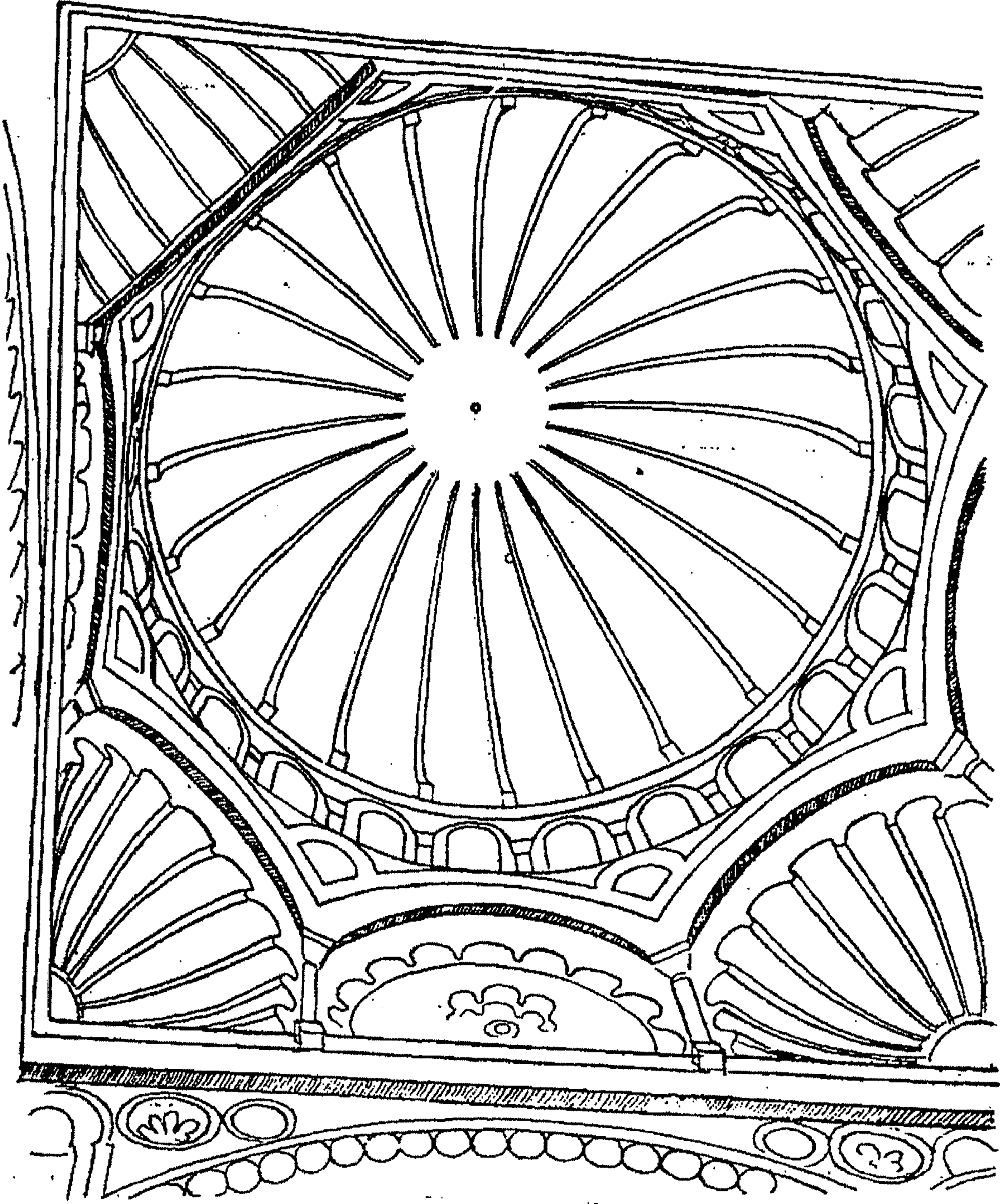
(شكل رقم ١٧) رسم تحليلي لهيكل قبة المحراب بجامع القيروان عن د/ أحمد فكري
